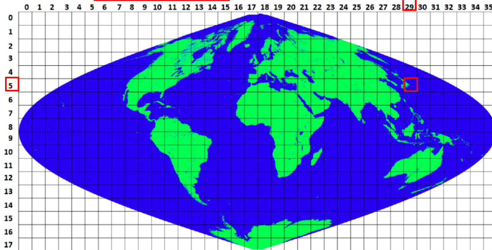
図 4-6 EQA (sinusoidal equal area) 図法
